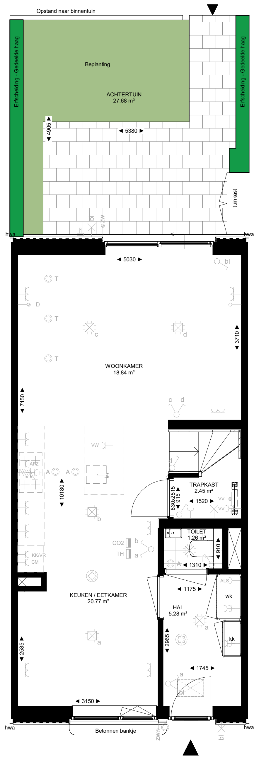
Begane grond
