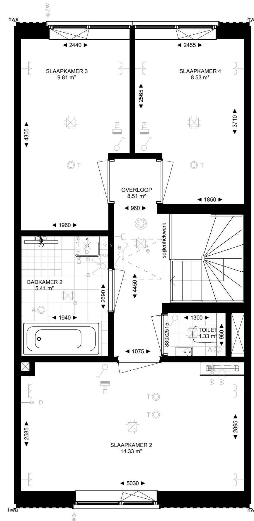
2e verdieping
