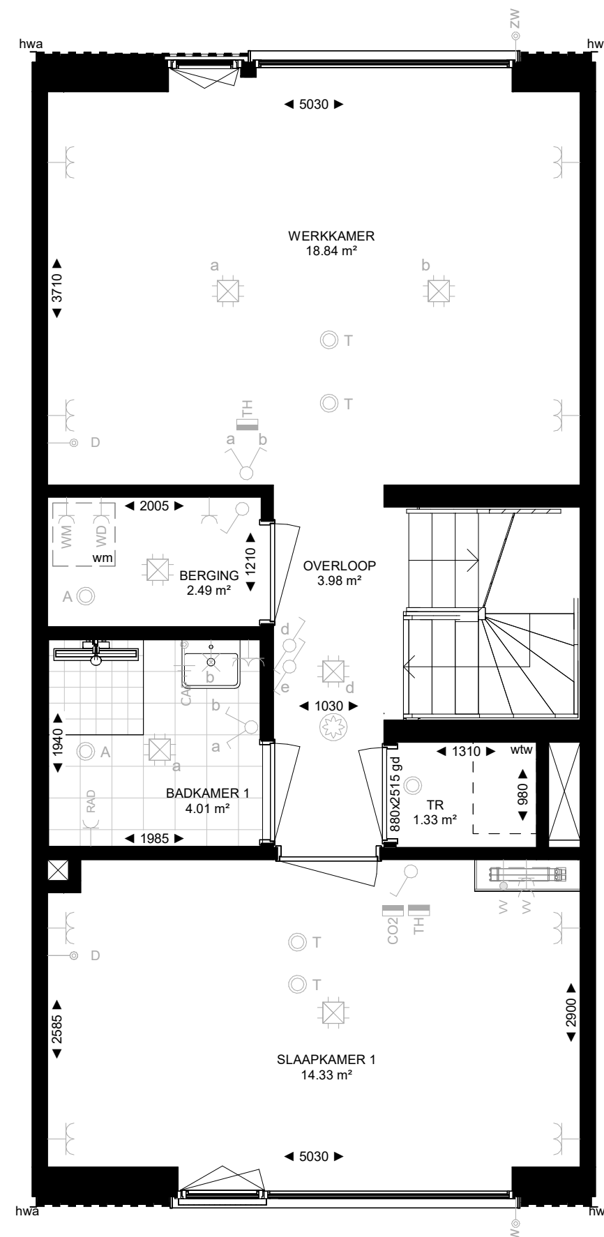
1e verdieping
